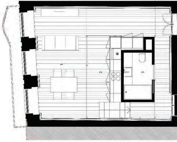
Planta Piso 1
